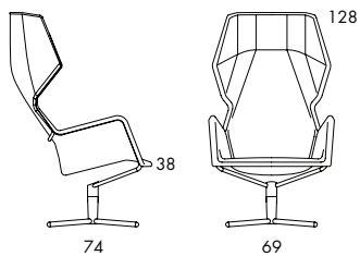
O43 10.6 kg | 0.85 m 3 /pc (1.45 m 3 /2 pcs)
